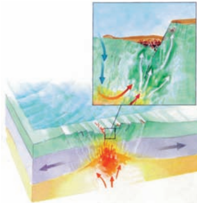
شکل ۶-۸- دگرگونی هیدروترمال ممکن است، در محل رشته‌کوه و سبب اقیانوس‌ها و به هنگام نفوذ آب سرد به داخل سنگ‌های بازالتی داغ موجب دگرسانی سنگ‌ها شود.
