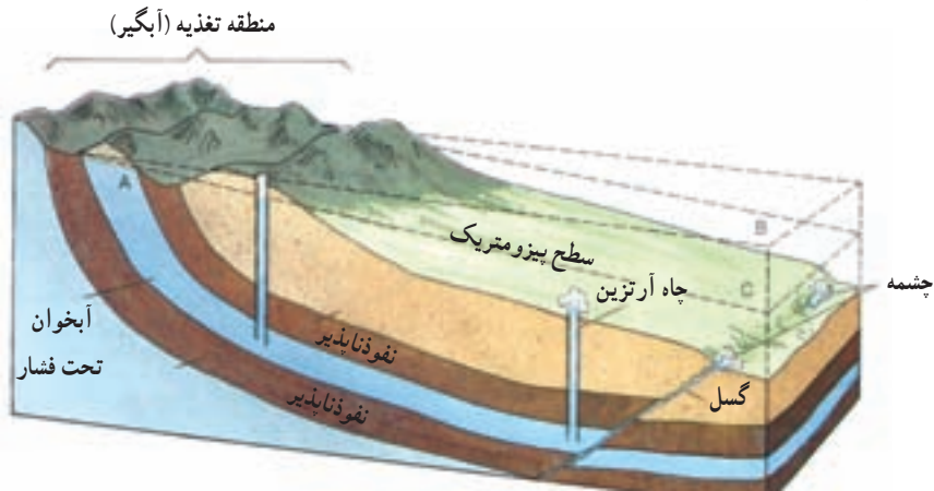
شكل ٧-٤- أبخوان تحت فشار
