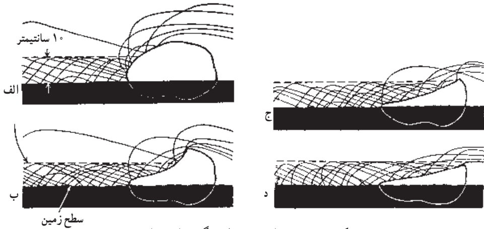
شکل ۹-۱۵ ذرات ماسه سطح سنگ ها را می خراشند.
